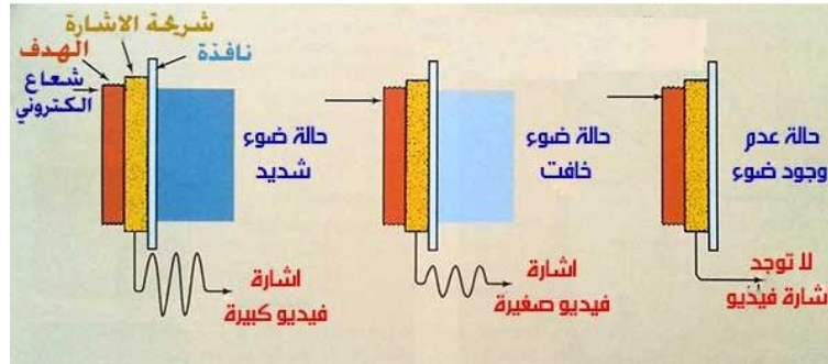
الشكل 3-2 علاقة سعة إشارة الصورة مع شدة الضوء الساقط
