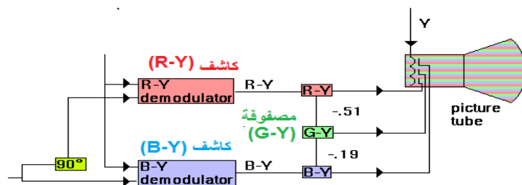
الشكل 2-5 مصفوفة (G-Y)
