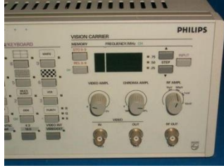
الشكل 2-1 بعض أشكال لأجهزة مولد النموذج
