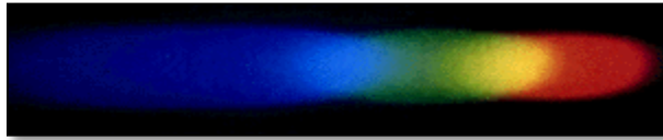
الشكل 1-1 ألوان الطيف الأبيض عند تحليلها
